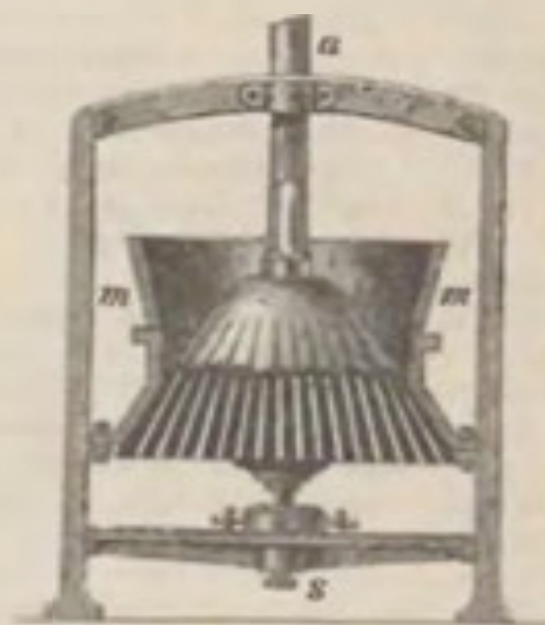
Obr. 132. Mlýn zvonový.
